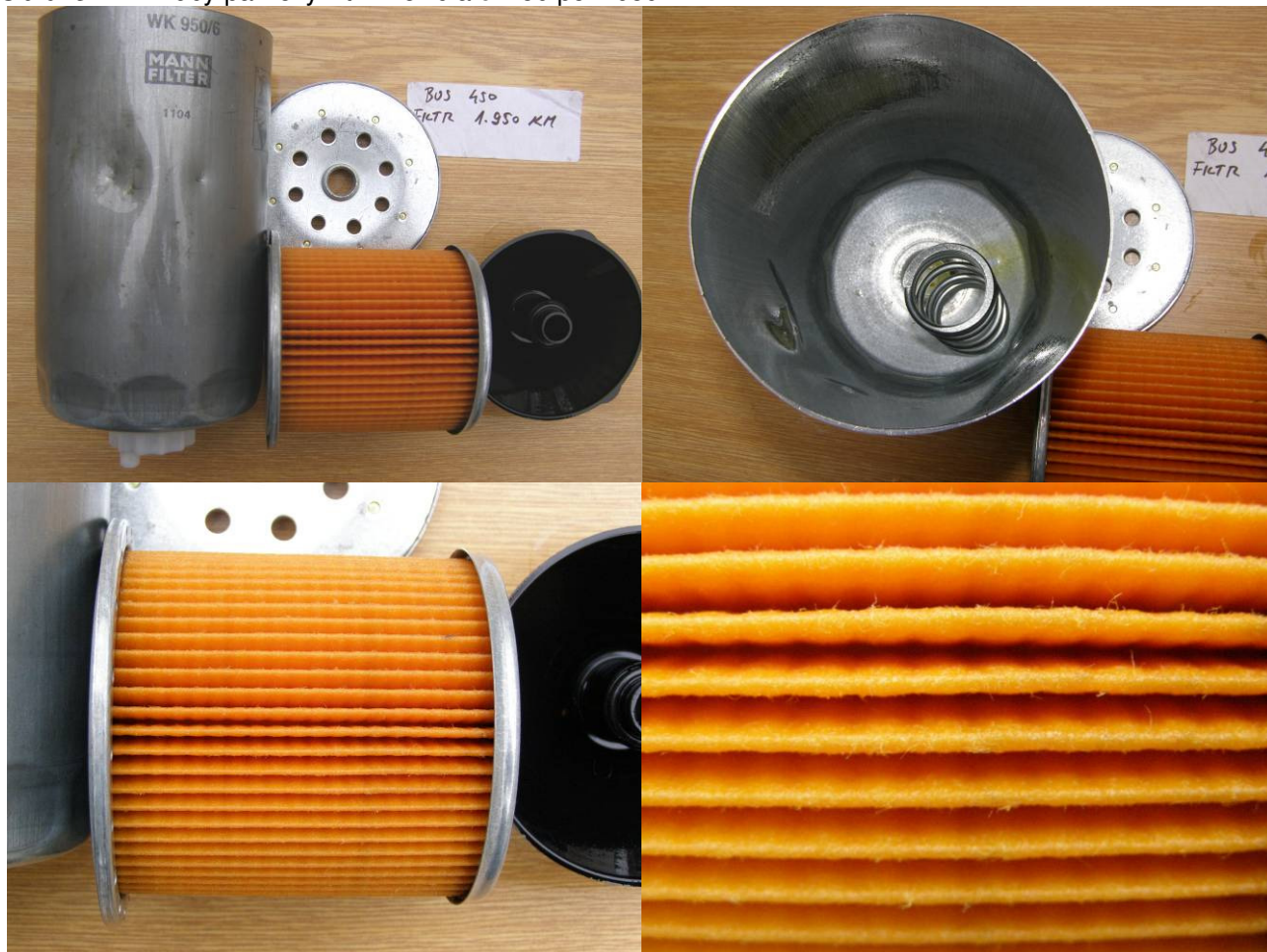
Obrázek 12 Předfiltr na sání paliva v nádrži autobusu SOR BN10.5
