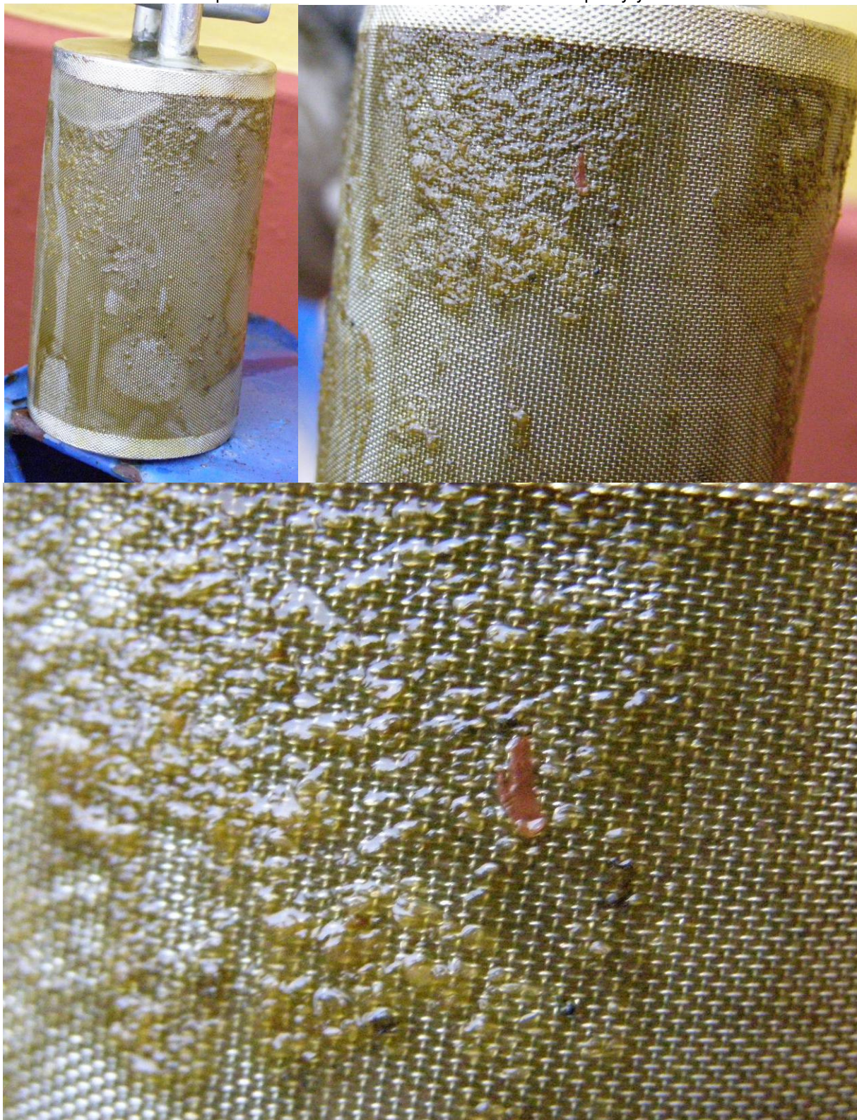
Obrázek 13 Předfiltr na sání paliva v nádrži autobusu SOR SOR BN10.5 pokrytý usazeninami
