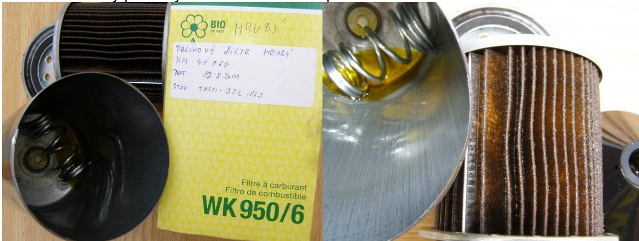
Obrázek 17 Hrubý palivový filtr z vozidla č. 603 po 41 067 km
