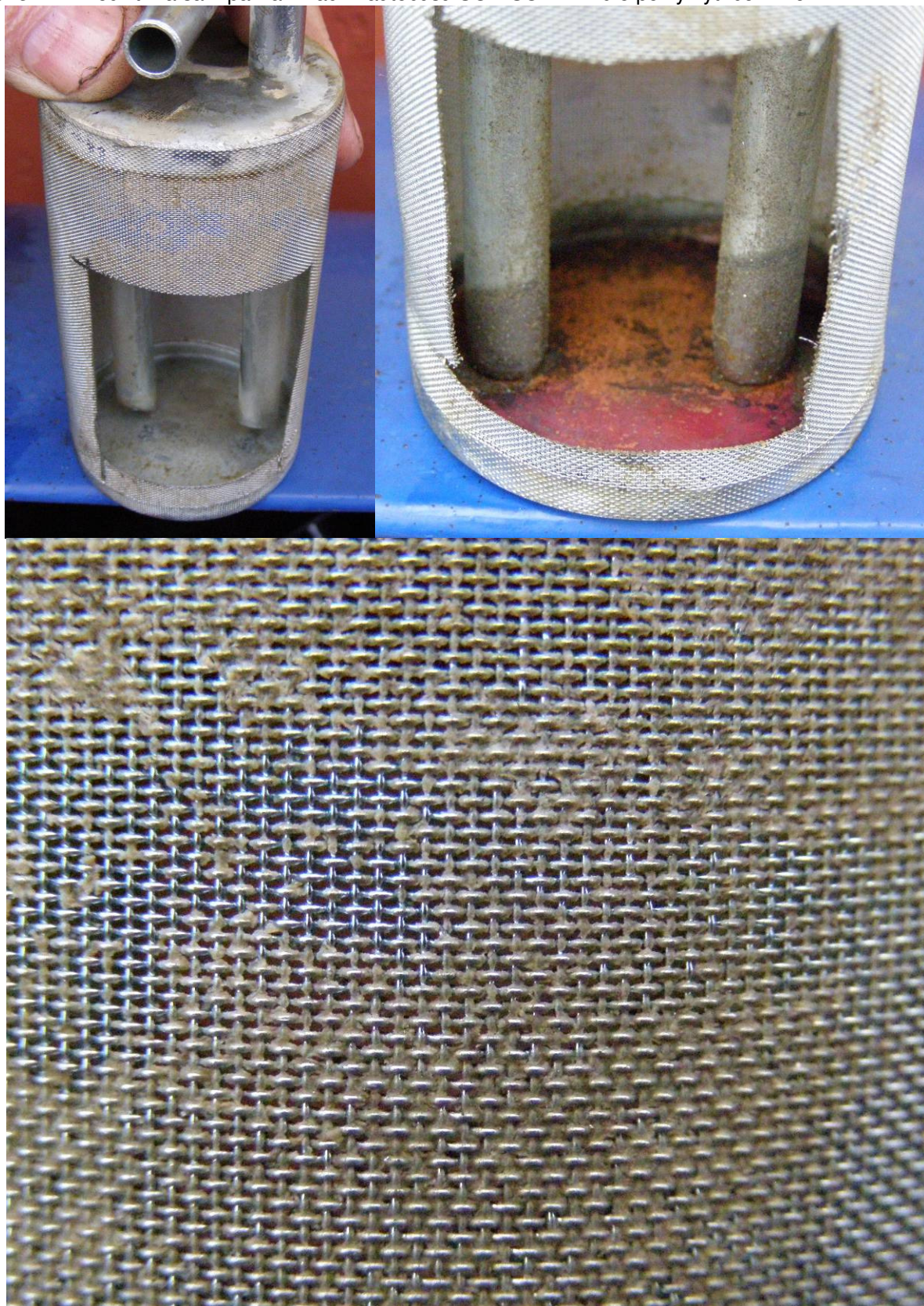
Obrázek 14 Předfiltr na sání paliva v nádrži autobusu SOR SOR BN10.5 po vymytí benzínem
