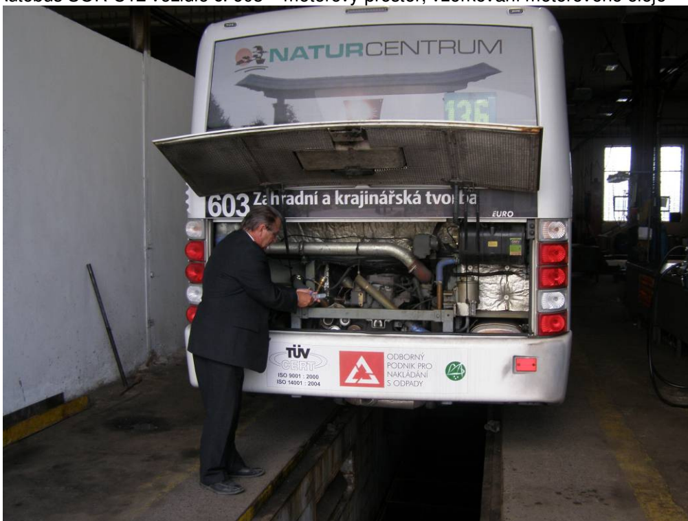
Obrázek 4 Autobus SOR C12 vozidlo č. 603 – motorový prostor, vzorkování motorového oleje
